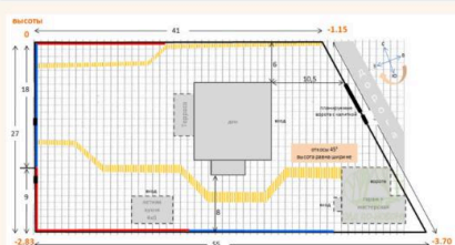
1. план исходной ситуации
